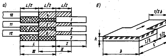
Рис. 27. Шахматная схема набора грунта.
