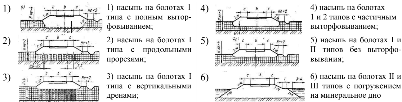
Рис. 46. Конструкции поперечных профилей земляного полотна на болотах.
