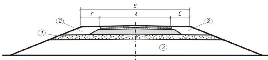
Рис. 60. Конструкция бескорытного поперечного профиля.
